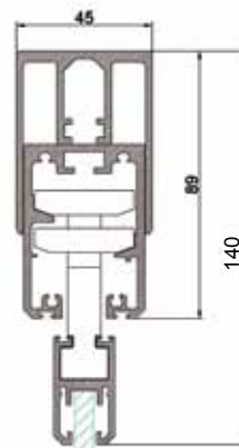
PERFIL GUÍA INFERIOR STANDARD
