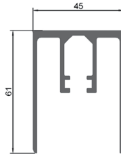
PERFIL HOJA 8MM STANDARD
