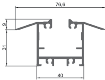
PERFIL GUÍA INFERIOR EMBUTIDA STANDARD
