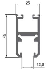
PERFIL HOJA 12MM STANDARD
