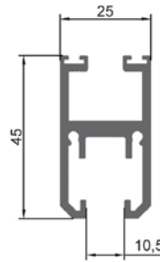
PERFIL HOJA 10MM STANDARD
