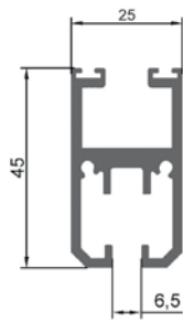
PERFIL GUÍA INFERIOR EMBUTIDA STANDARD
