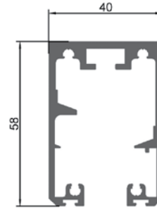
PERFIL GUÍA SUPERIOR STANDARD
