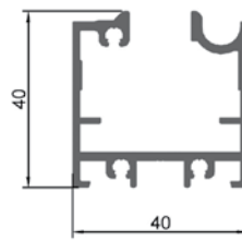
PERFIL GUÍA INFERIOR STANDARD
